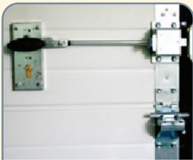
Option SCHLOSS mit Einsatz und 3 Schlüsseln
